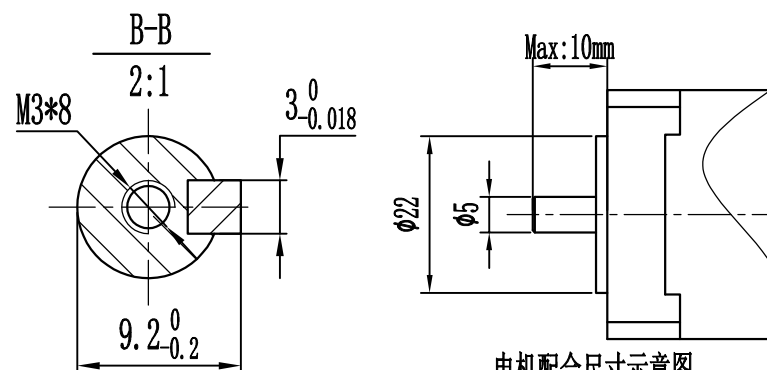
电机配合尺寸示意图 Motor size
