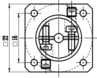
输入端Input
