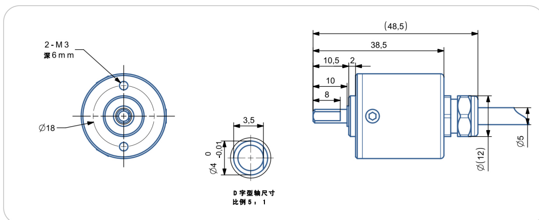
尺寸型号图6: 输出轴4mm尾出 IP54 (此尺寸编码器分辨率可选: 1024、4096、16384、32768)
