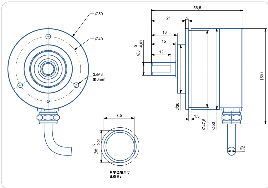
尺寸型号图12：输出轴8mm IP68/防爆
