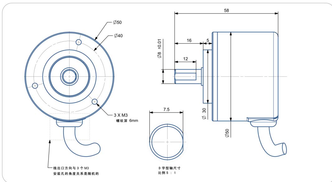
尺寸型号图5: YL50输出轴10mm IP54
