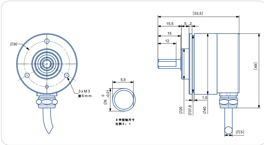
尺寸型号图8: 输出轴6mm IP68/防爆
