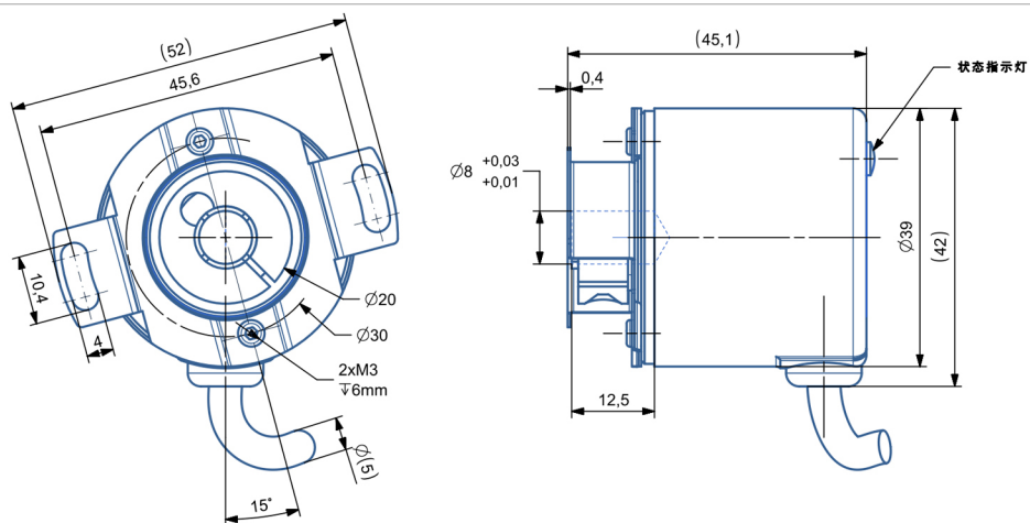
尺寸型号图3: 抱箍8mm IP54
