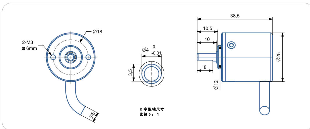
尺寸型号图7: 输出轴4mm侧出 IP54 (此尺寸编码器分辨率可选: 1024、4096、16384、32768)
