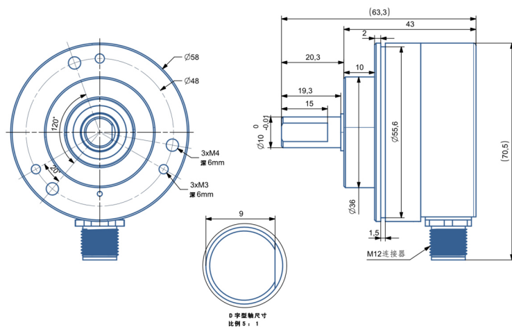
尺寸型号图14: 输出轴10mm IP68/防爆
