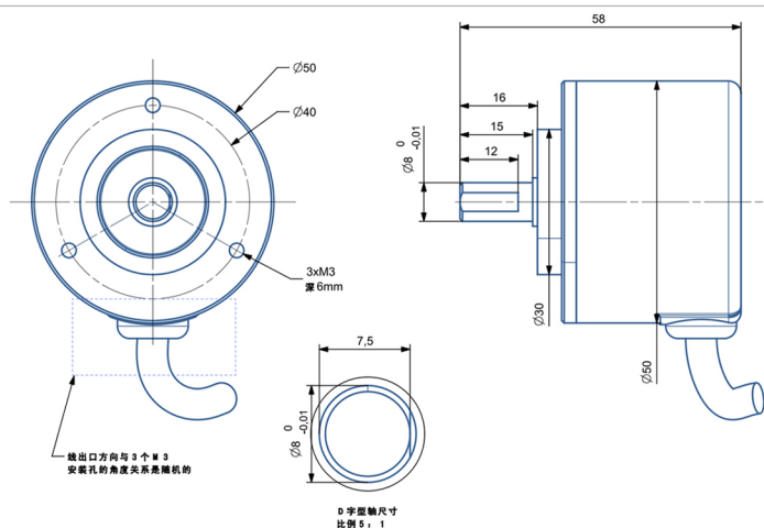
尺寸型号图3: 抱箍8mm IP54
