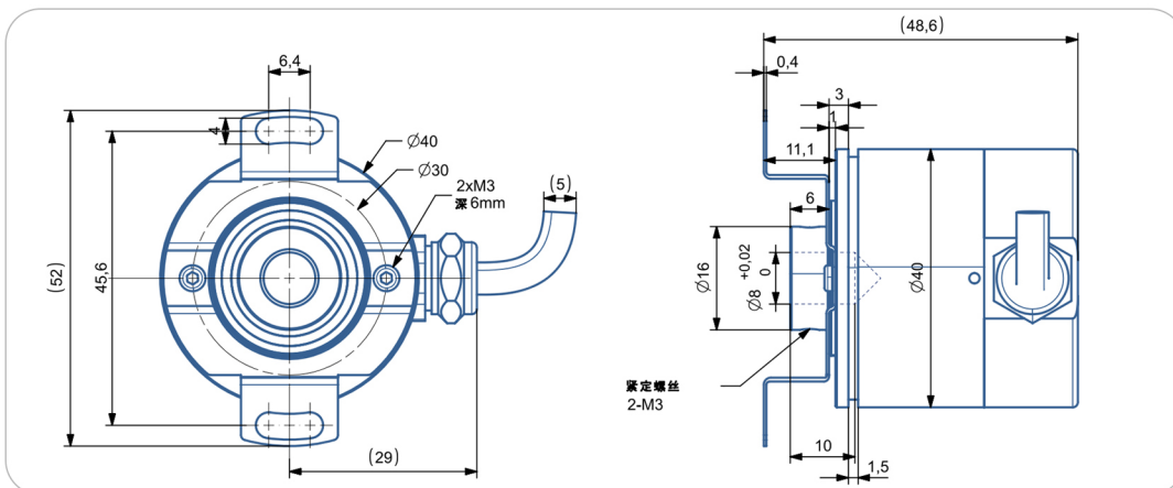
尺寸型号图10: 输出轴8mm盲孔 IP68/防爆
