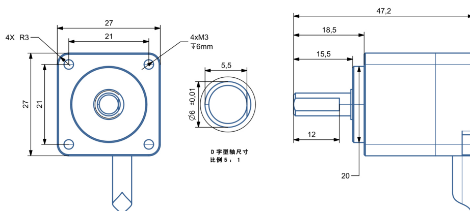
尺寸型号图13: 输出轴6mm IP68/防爆
