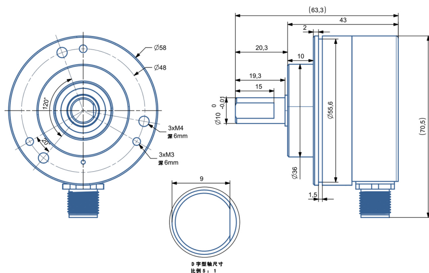
尺寸型号图12: 输出轴10mm IP68/防爆
