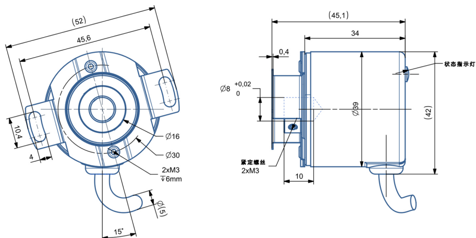
尺寸型号图2: 盲孔8mm IP54
