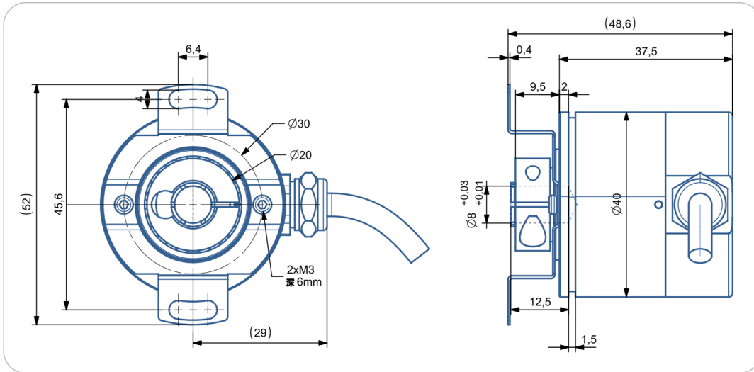
尺寸型号图11：抱箍8mm IP68/防爆
