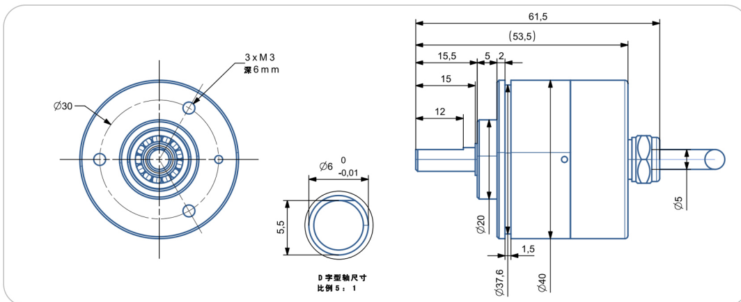
尺寸型号图9: 输出轴6mm尾出 IP68/防爆
