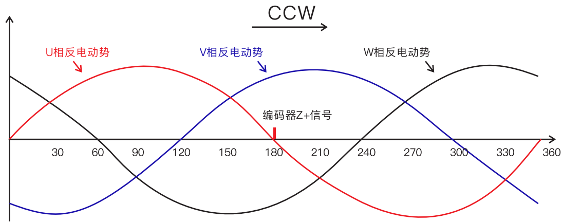
编码器零点与电机相位关系
