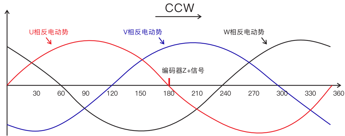
编码器零点与电机相位关系
