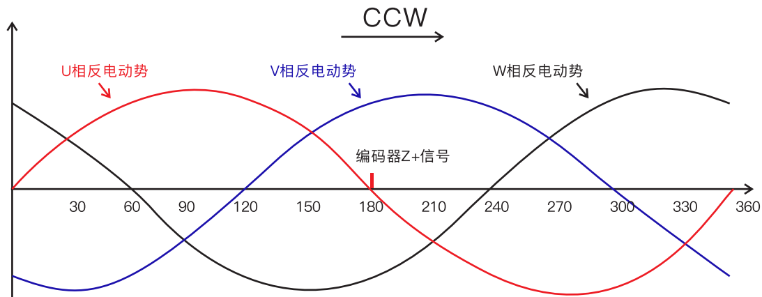
编码器零点与电机相位关系
